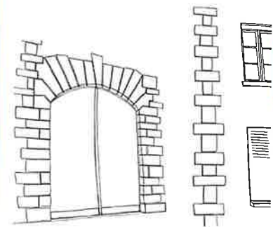
Encadrement d'un porche et harpe en pierre de taille
