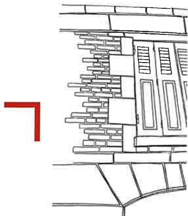
Corniche, bandeau, encadrements de fenêtre et de porche en pierre de taille sur une façade en brique
