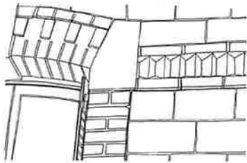
Encadrement, linteau en brique et pierre de taille, bandeau avec dents d'engrenage (rang de brique saillante disposée en biais)
