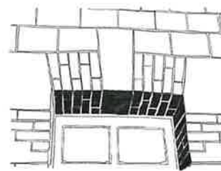
Les linteaux, corniches, tableaux des façades des maisons 19 ème sont souvent en brique
