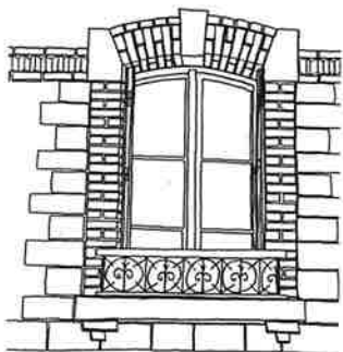
Ouverture avec encadrement en brique, linteau cintré, appui en pierre et garde-corps en fonte
